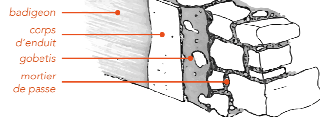
Coupe d'un mur de pierres avec les différentes utilisations de la chaux
